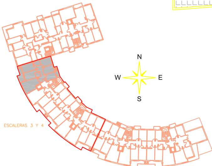
PLANTA TIPO (1 a a 4 a ). VIVIENDA TIPO B. HENS - PARCELA 4. ESCALERA 3
