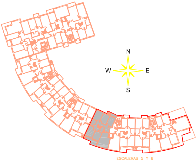
PLANTA QUINTA. VIVIENDA TIPO B. HENS - PARCELA 4. ESCALERA 5
