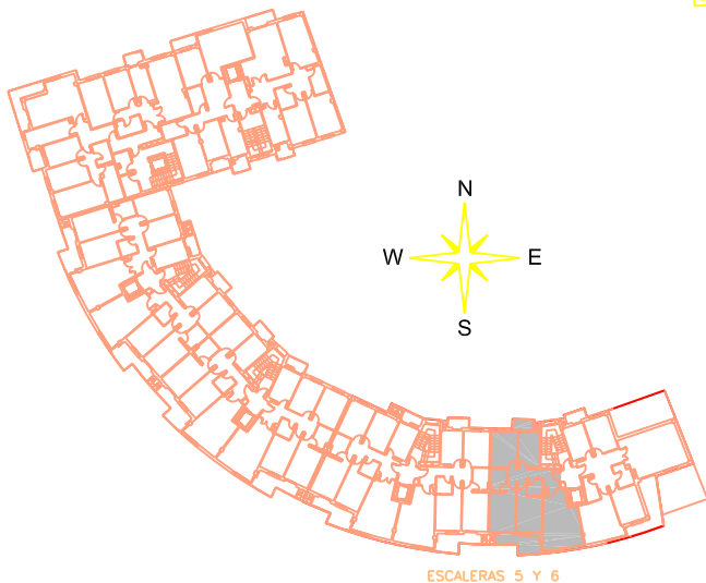
PLANTA PRIMERA. VIVIENDA TIPO B. HENS - PARCELA 4. ESCALERA 6
